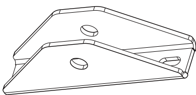
Torbefestigungswinkel (×2)
